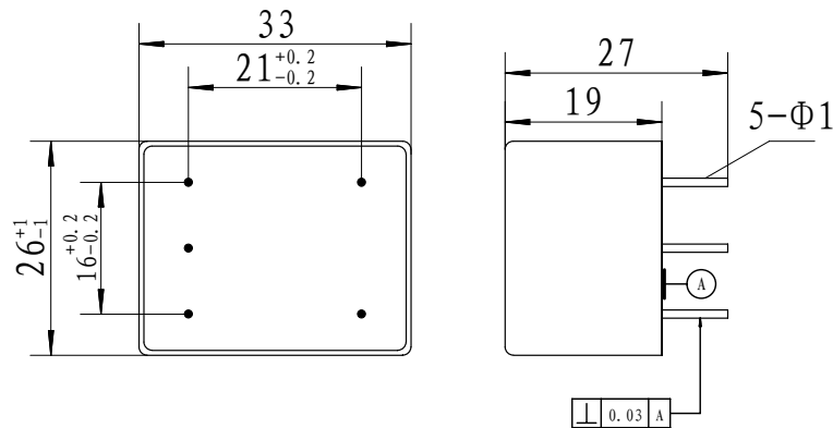
外形尺寸图
